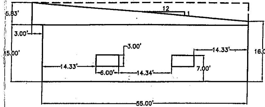
N.E. ELEVATION SCALE: 1" = 16'
