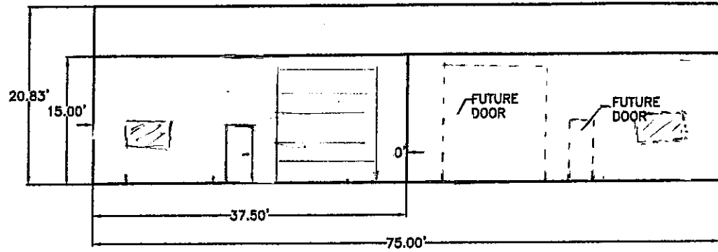
S.E. ELEVATION SCALE: 1" = 16'
